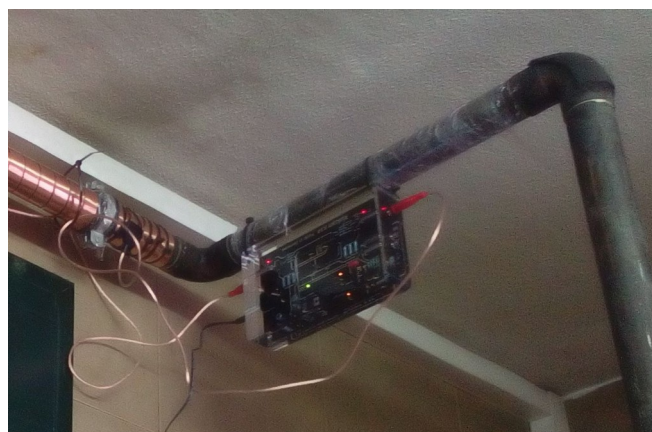
Vulcan S 10 - Heisswasser Kreislauf
