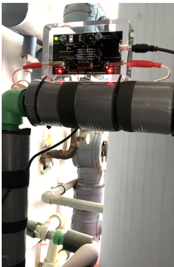
Vulcan 5000 Heiswasser Kreislauf mit Ø 32 mm
